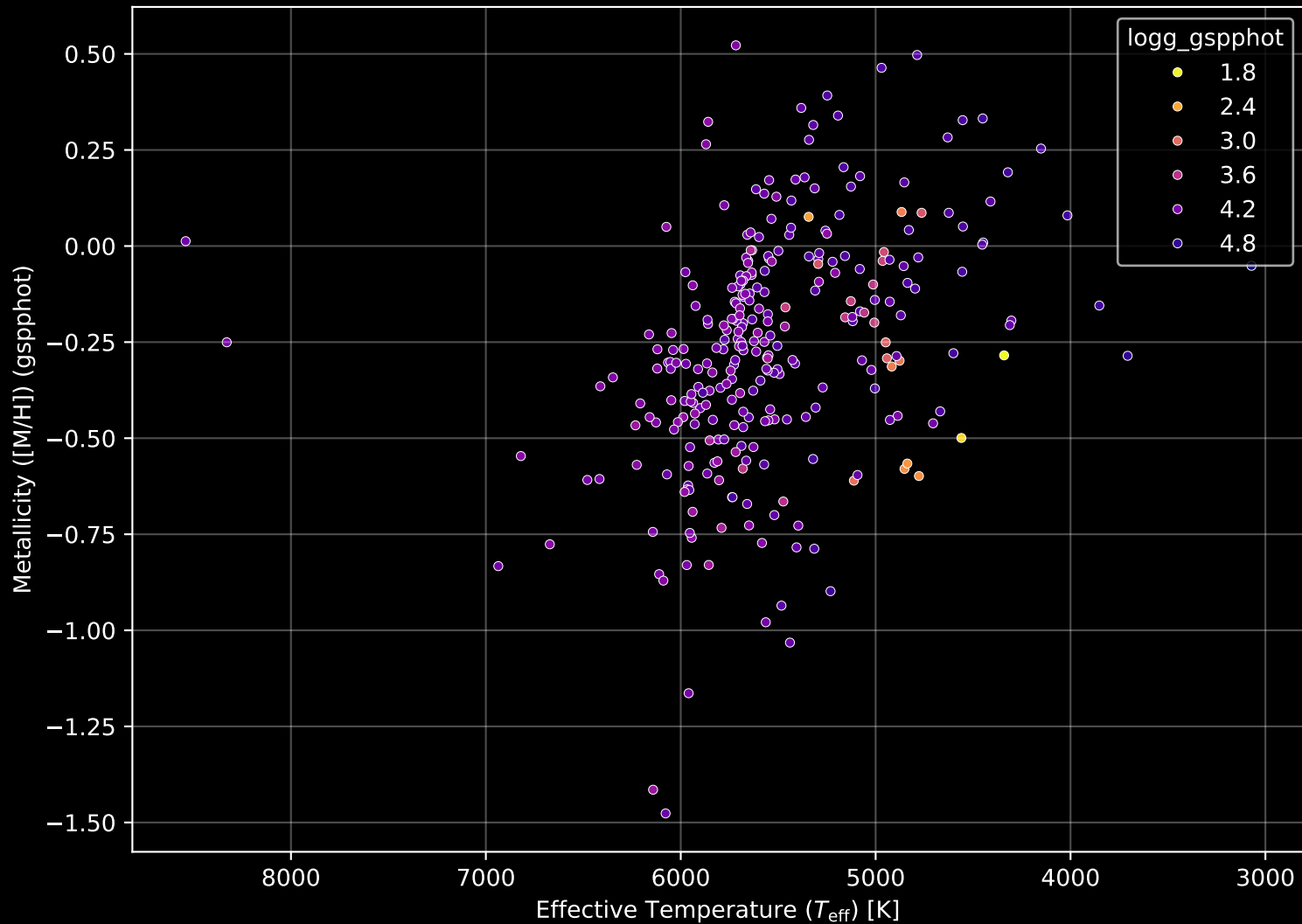
GALAH DR4 Field: [6925] Stellar Population Parameters (n= 288)
