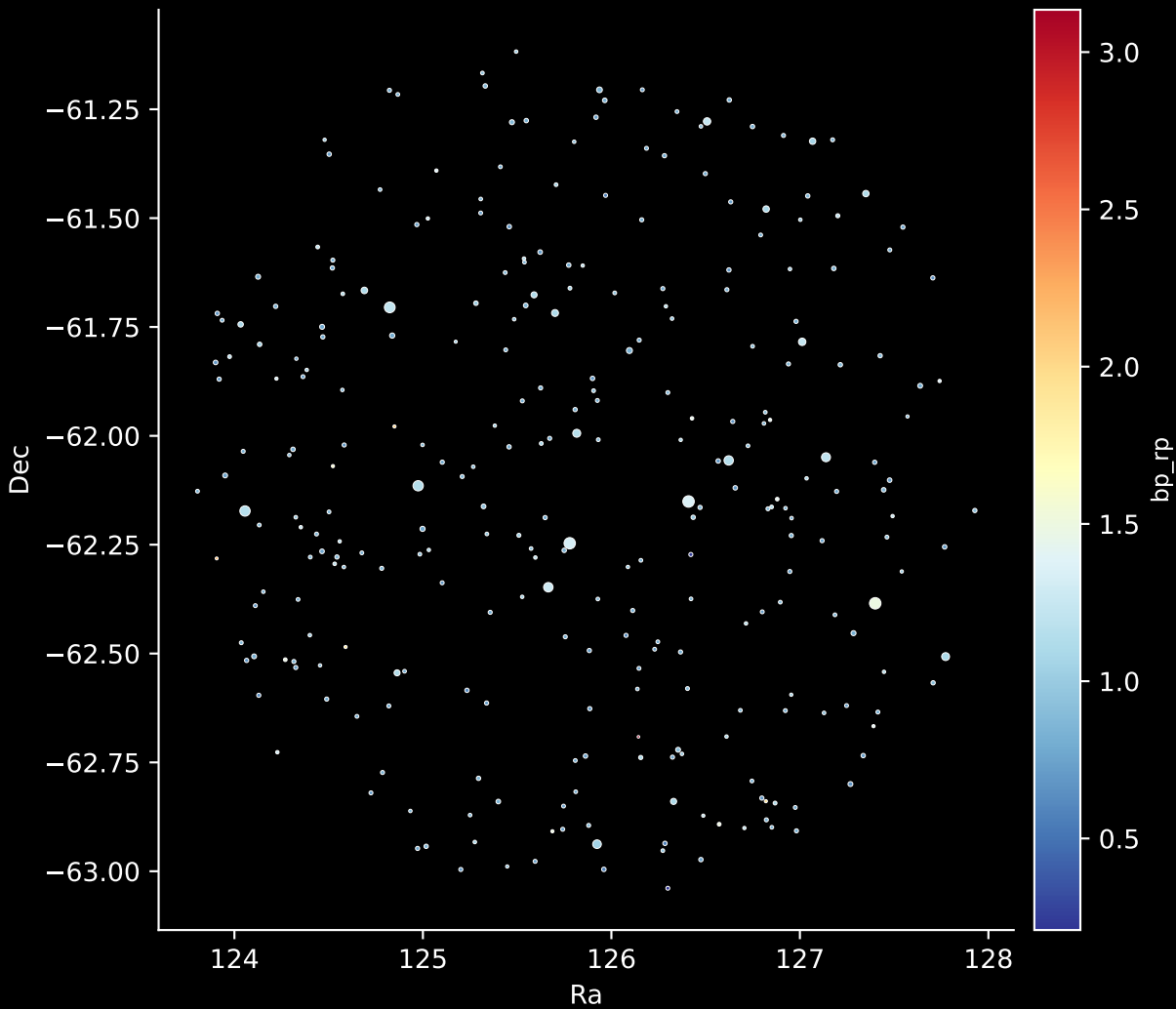
GALAH DR4 Field: [6925] Stars: 288
