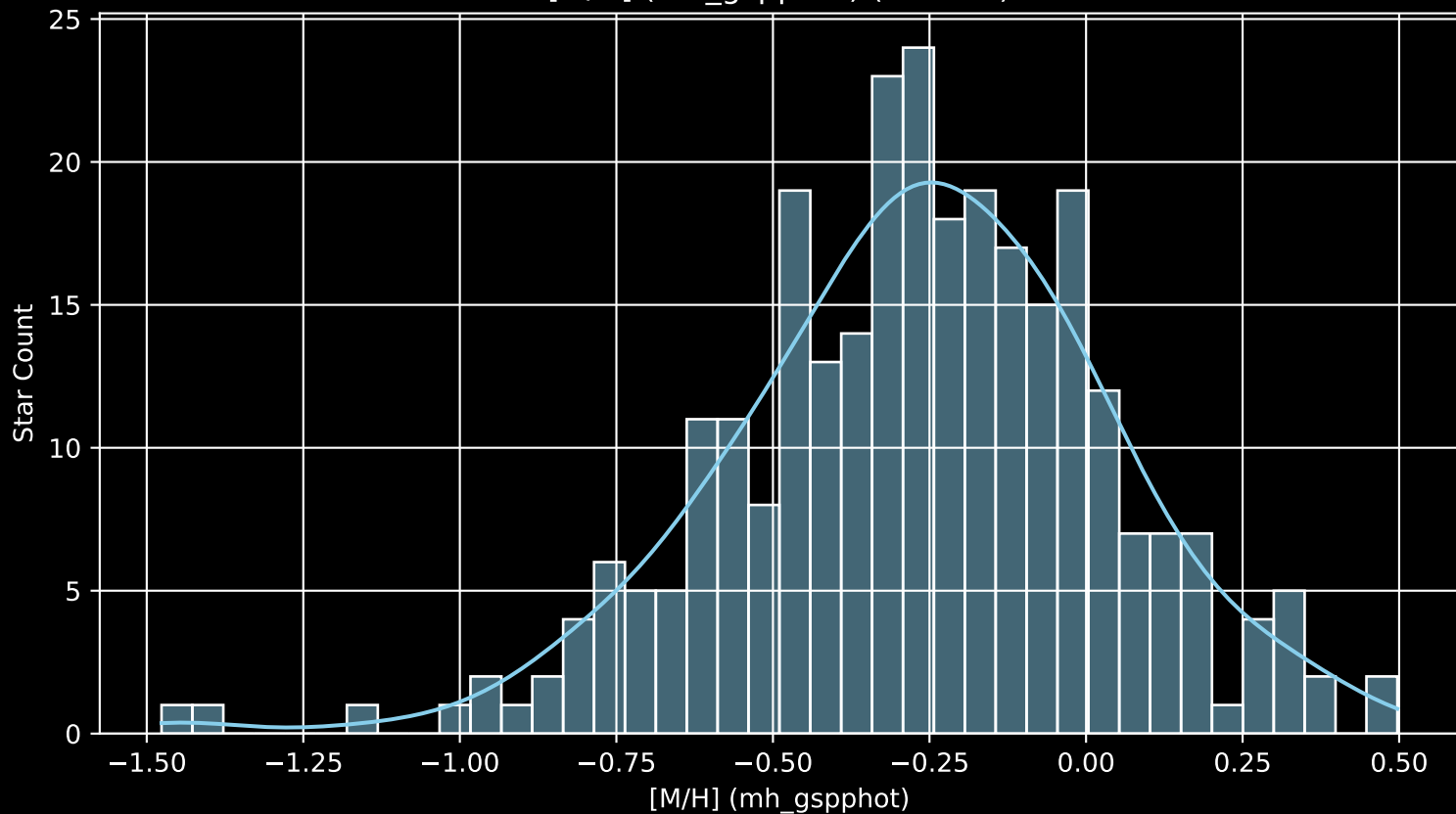
GALAH DR4 Field: [6925] [M/H] (mh_gspphot) (n= 287)
